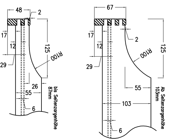
Englischer Zug geschweift
